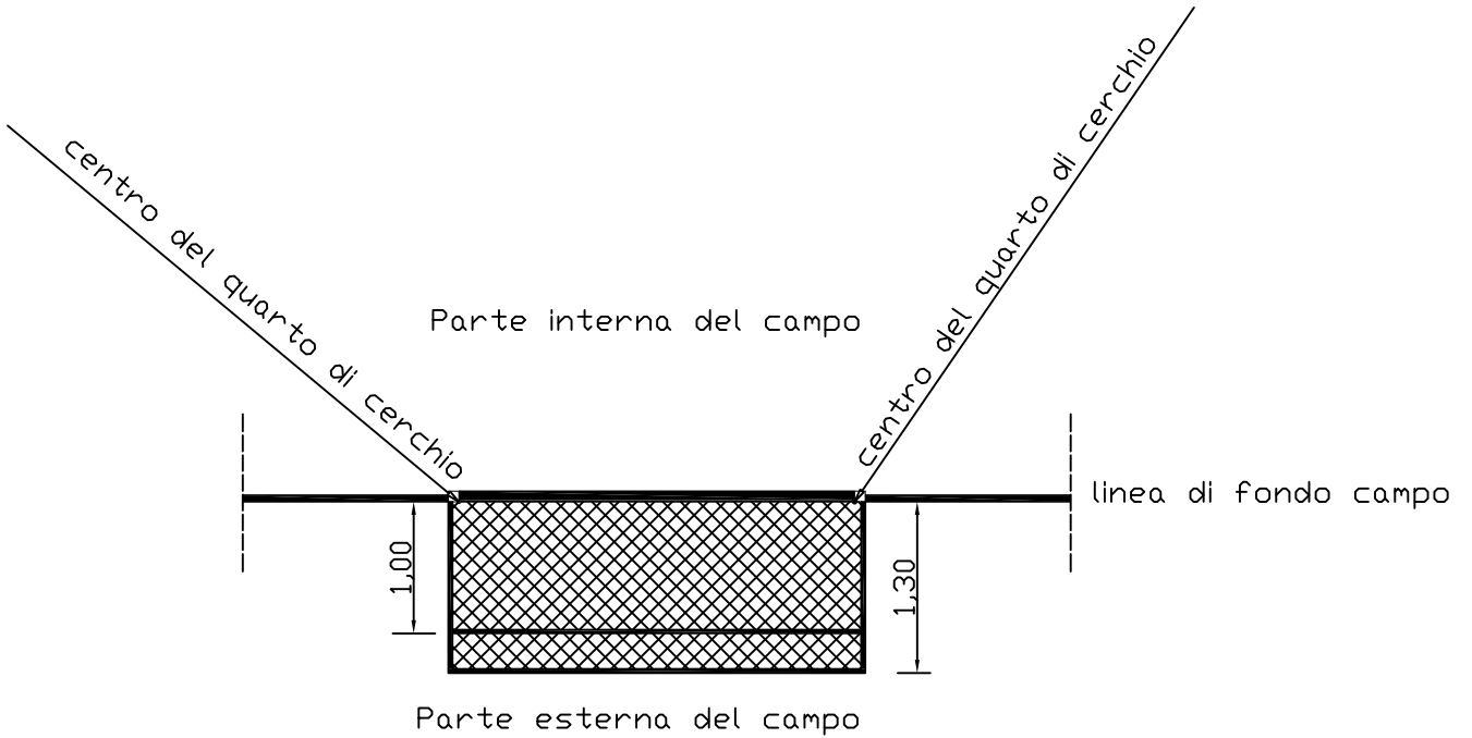
Pianta porta pallamano
