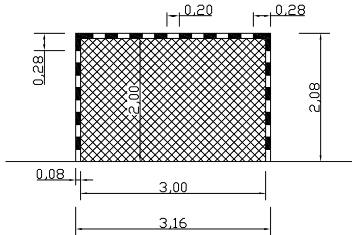
Prospetto porta pallamano
